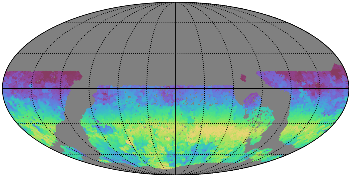
too_ignore_5_4v3.4_10yrs WFD y band: AngleRange rotSkyPos
