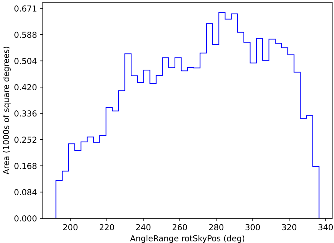
too_ignore_5_4v3.4_10yrs WFD y band: AngleRange rotSkyPos
