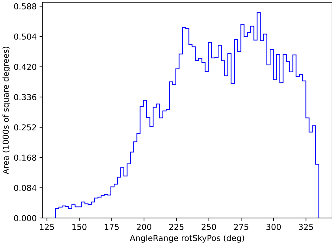
too_ignore_5_4v3.4_10yrs All sky y band: AngleRange rotSkyPos
