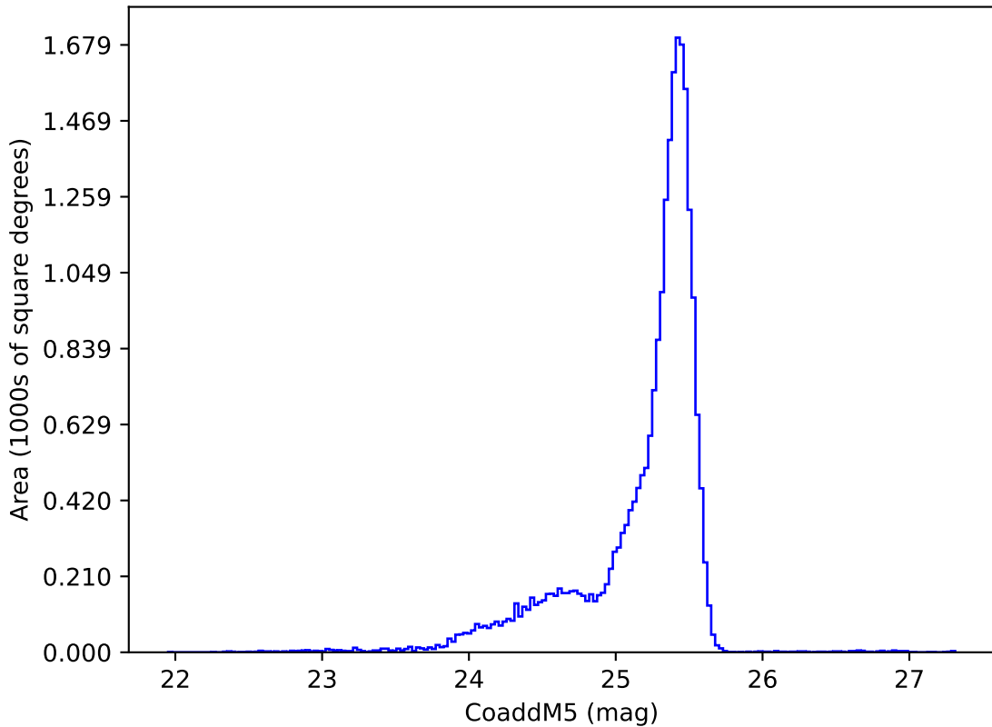
too_ignore_5_4v3.4_10yrs u: CoaddM5
