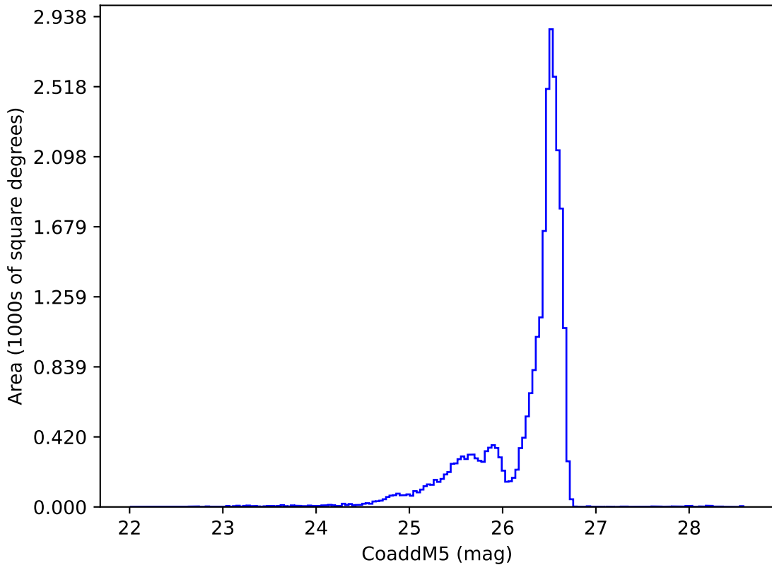
too_ignore_5_4v3.4_10yrs i: CoaddM5
