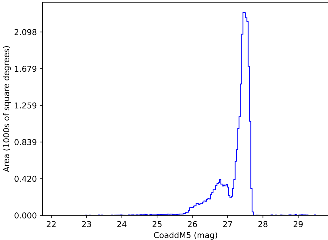
too_ignore_5_4v3.4_10yrs : CoaddM5
