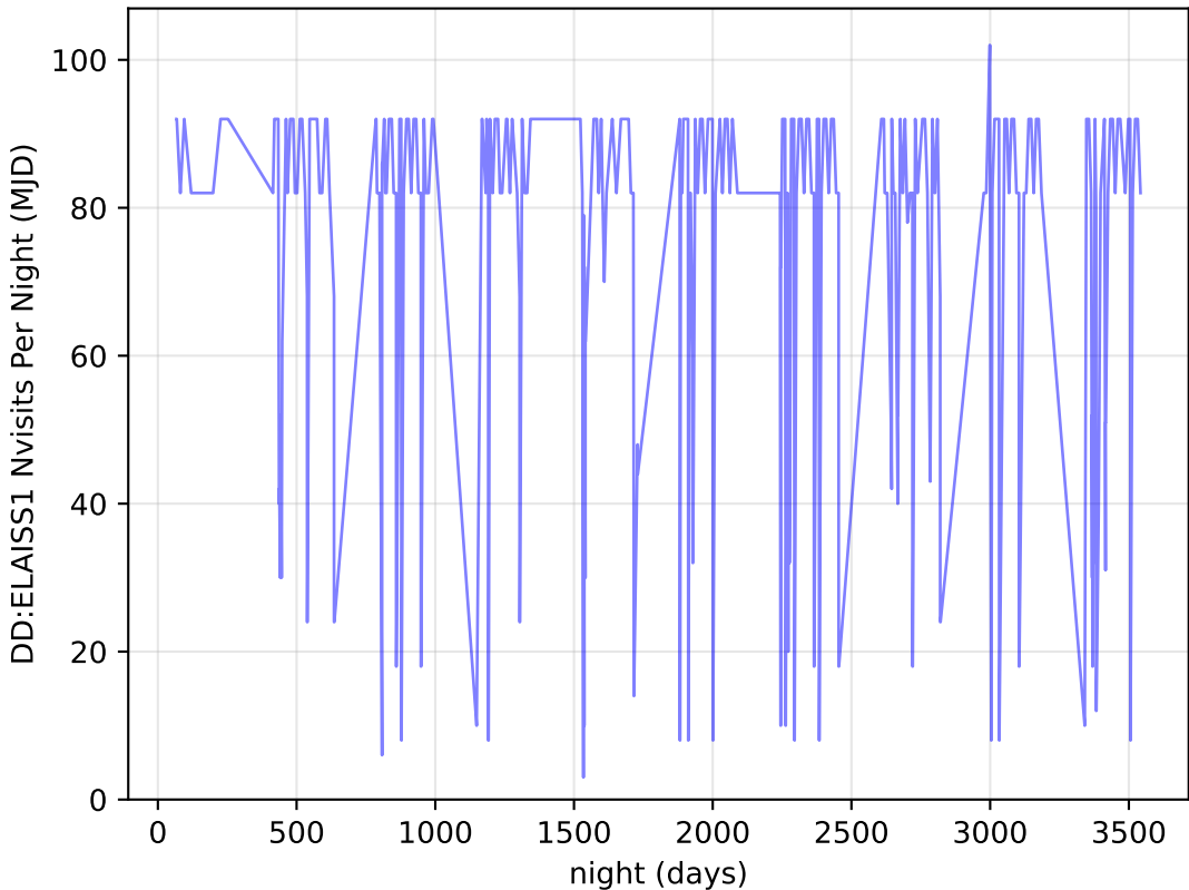
too_ignore_5_4v3.4_10yrs all bands: DD:ELAISS1 Nvisits Per Night
