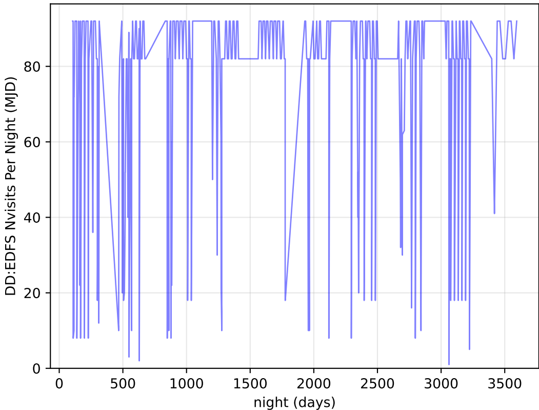
too_ignore_5_4v3.4_10yrs all bands: DD:EDFS Nvisits Per Night
