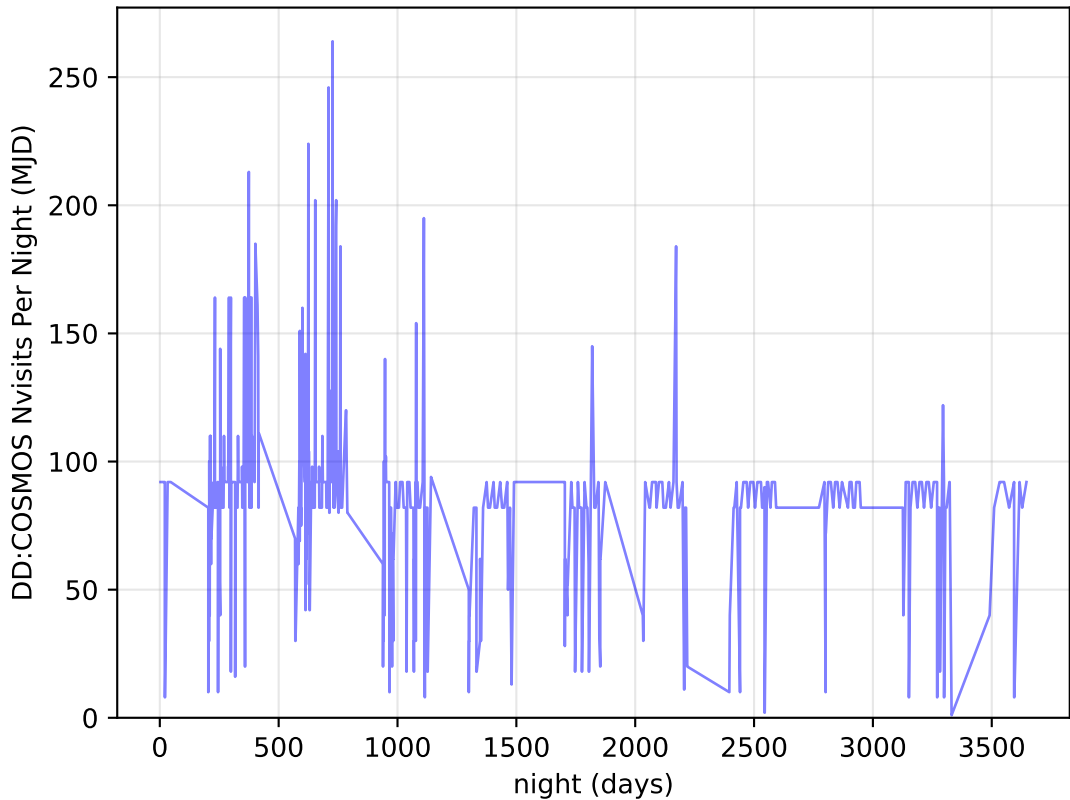
too_ignore_5_4v3.4_10yrs all bands: DD: COSMOS Nvisits Per Night
