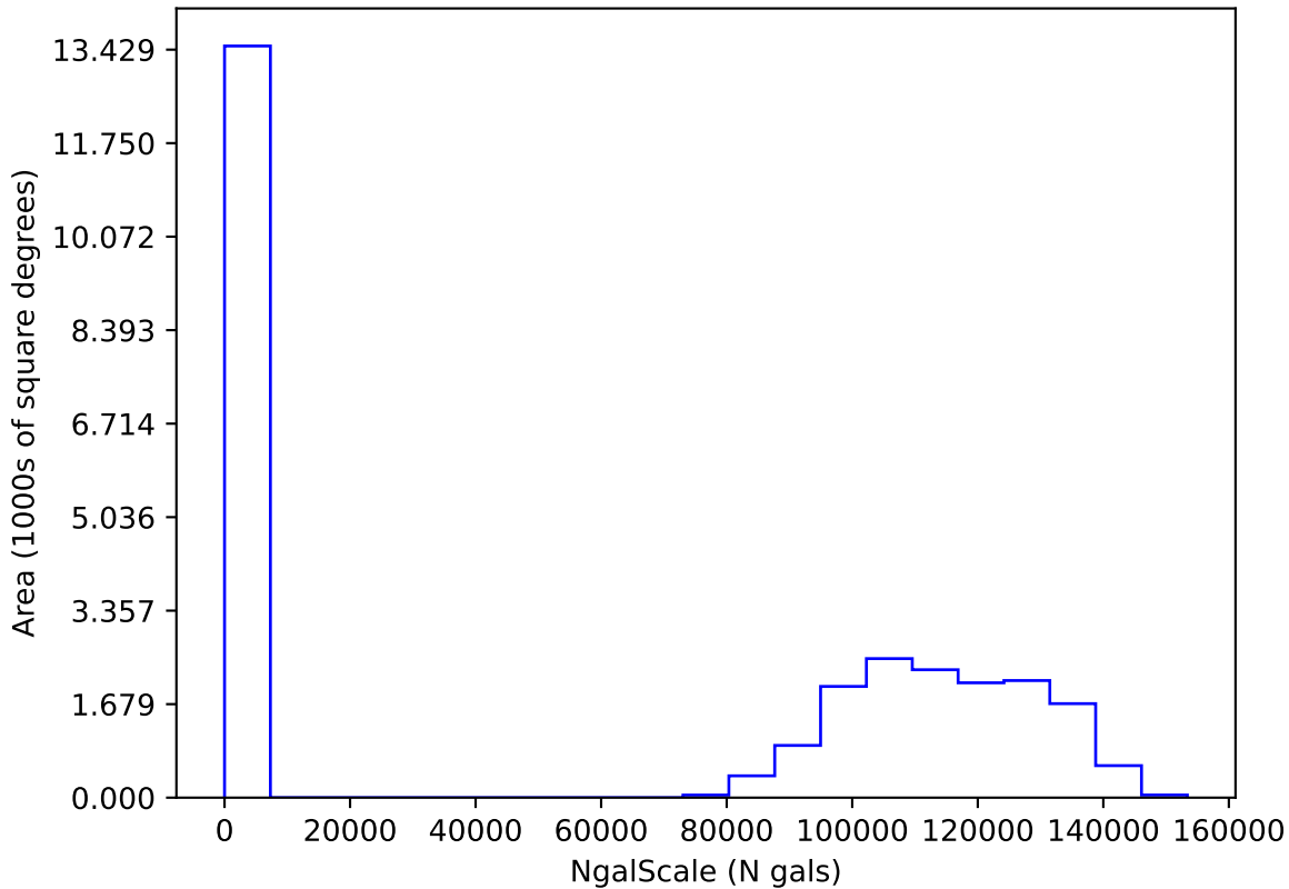
too_ignore_5_1v3.4_10yrs i: NgalScale
