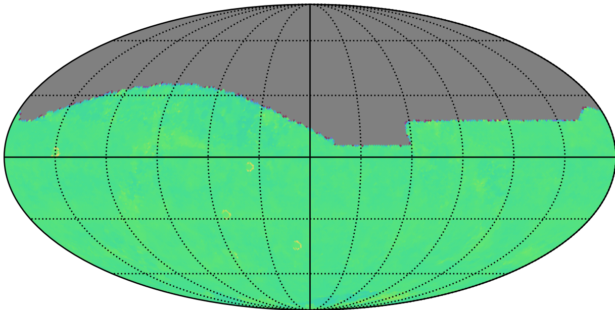
too_ignore_5_1v3.4_10yrs z: Kuiper rotTelPos
