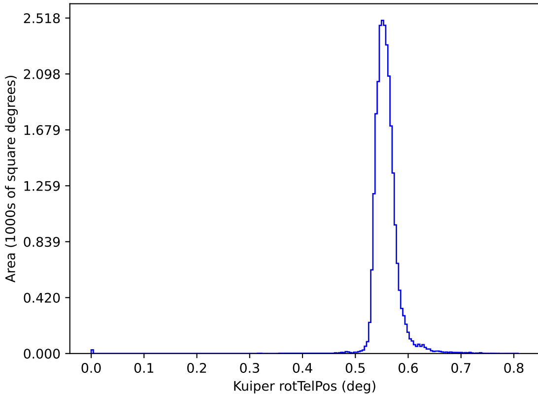
too_ignore_5_1v3.4_10yrs y: Kuiper rotTelPos
