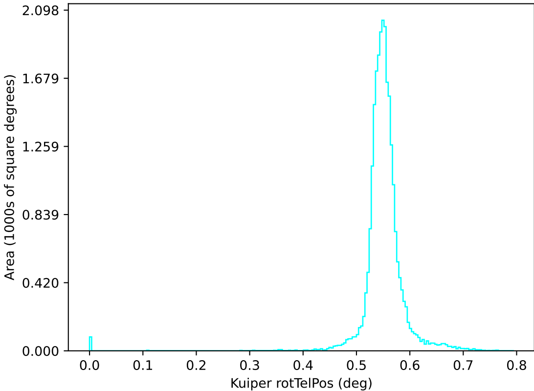
too_ignore_5_1v3.4_10yrs u: Kuiper rotTelPos
