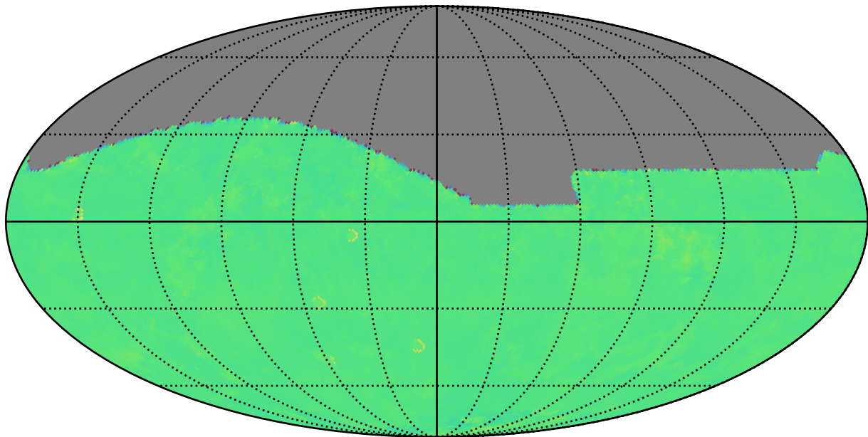
too_ignore_5_1v3.4_10yrs i: Kuiper rotTelPos
