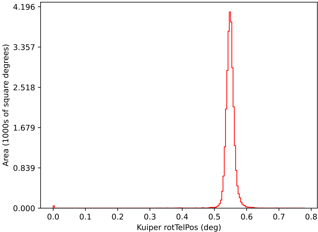
too_ignore_5_1v3.4_10yrs i: Kuiper rotTelPos
