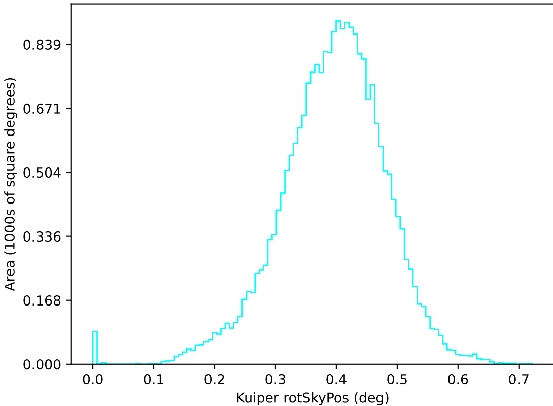
too_ignore_5_1v3.4_10yrs u: Kuiper rotSkyPos
