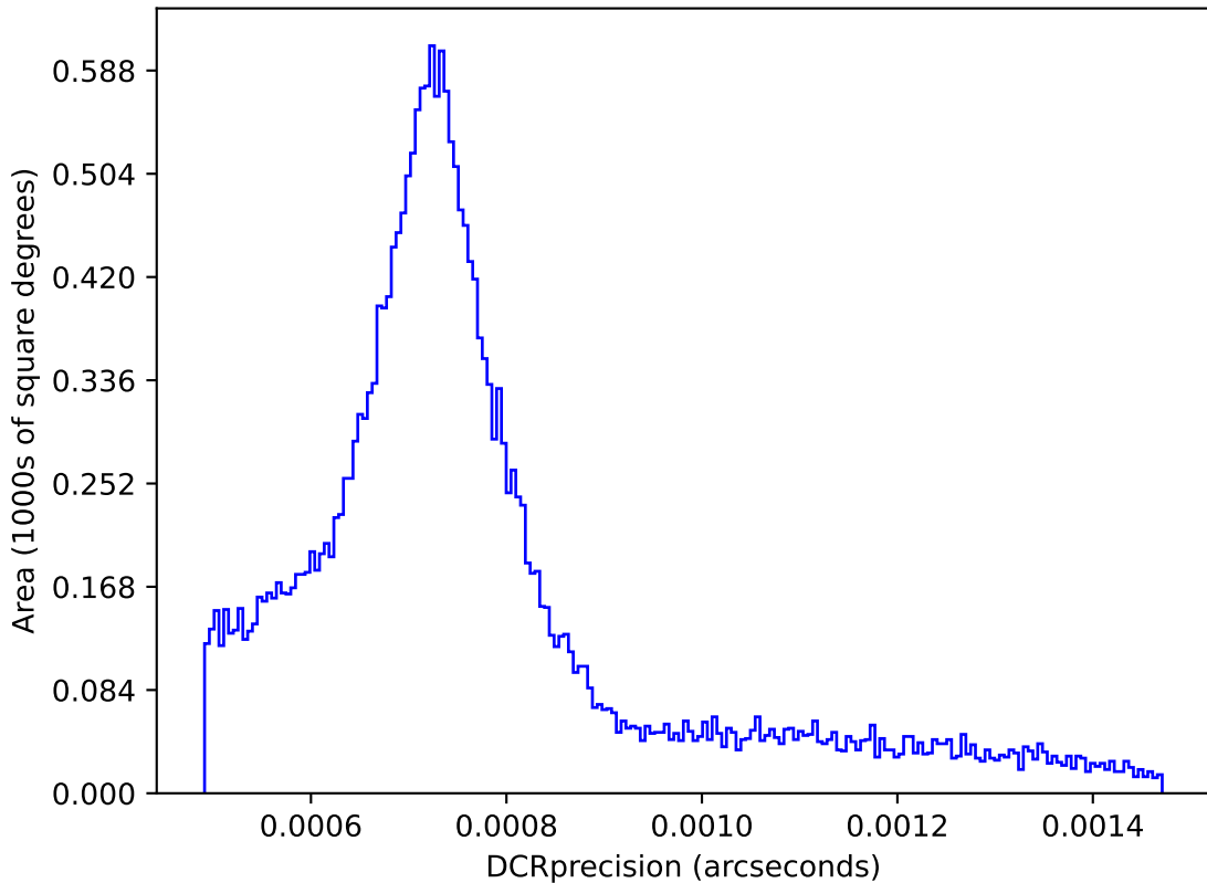
too_ignore_5_1v3.4_10yrs : DCRprecision
