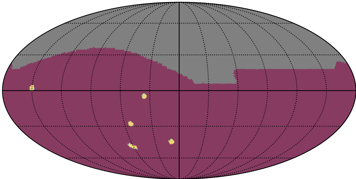
too_ignore_5_1v3.4_10yrs All sky: NumberOfQuickRevisits
