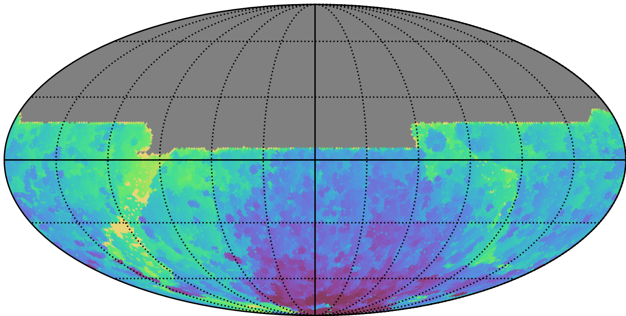
too_ignore_5_1v3.4_10yrs All sky y band: Min HA
