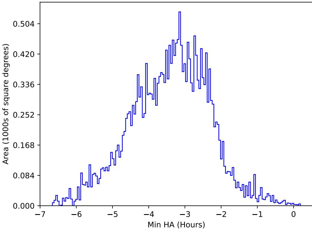
too_ignore_5_1v3.4_10yrs All sky y band: Min HA
