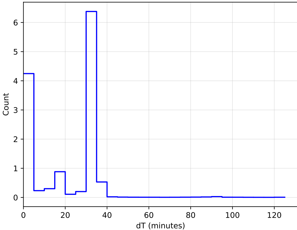
1e6 too_ignore_5_1v3.4_10yrs All sky: DeltaT Histogram
