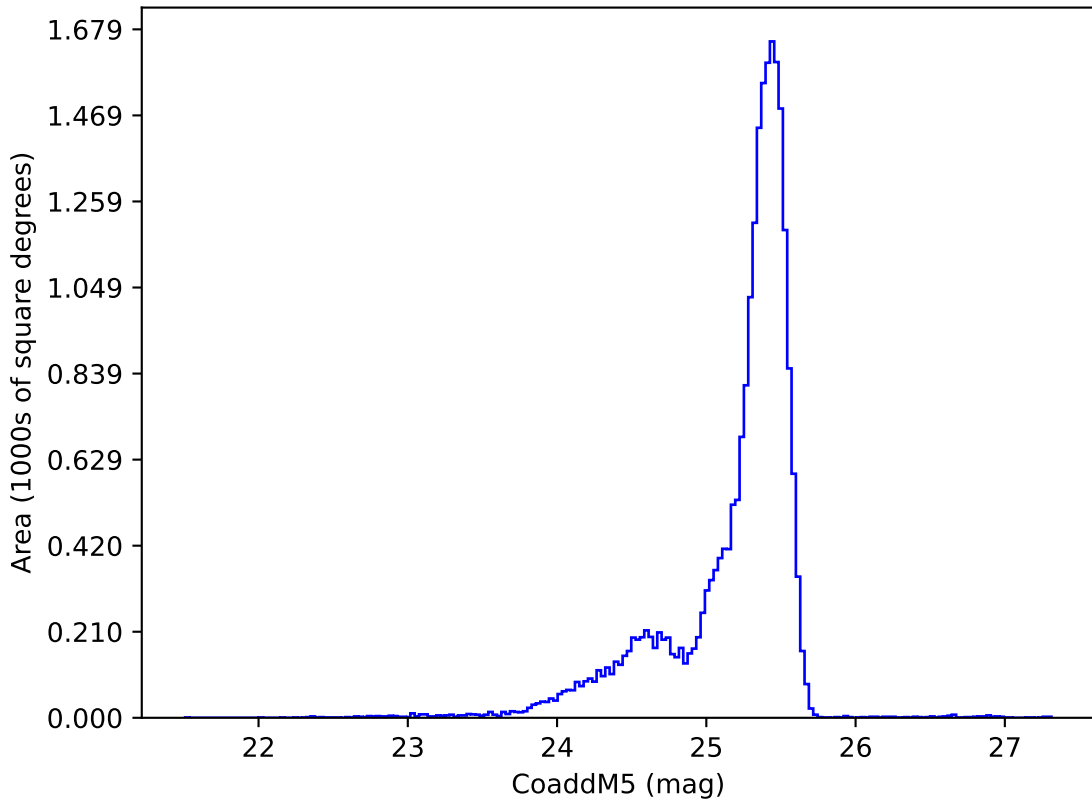
too_ignore_5_1v3.4_10yrs u: CoaddM5
