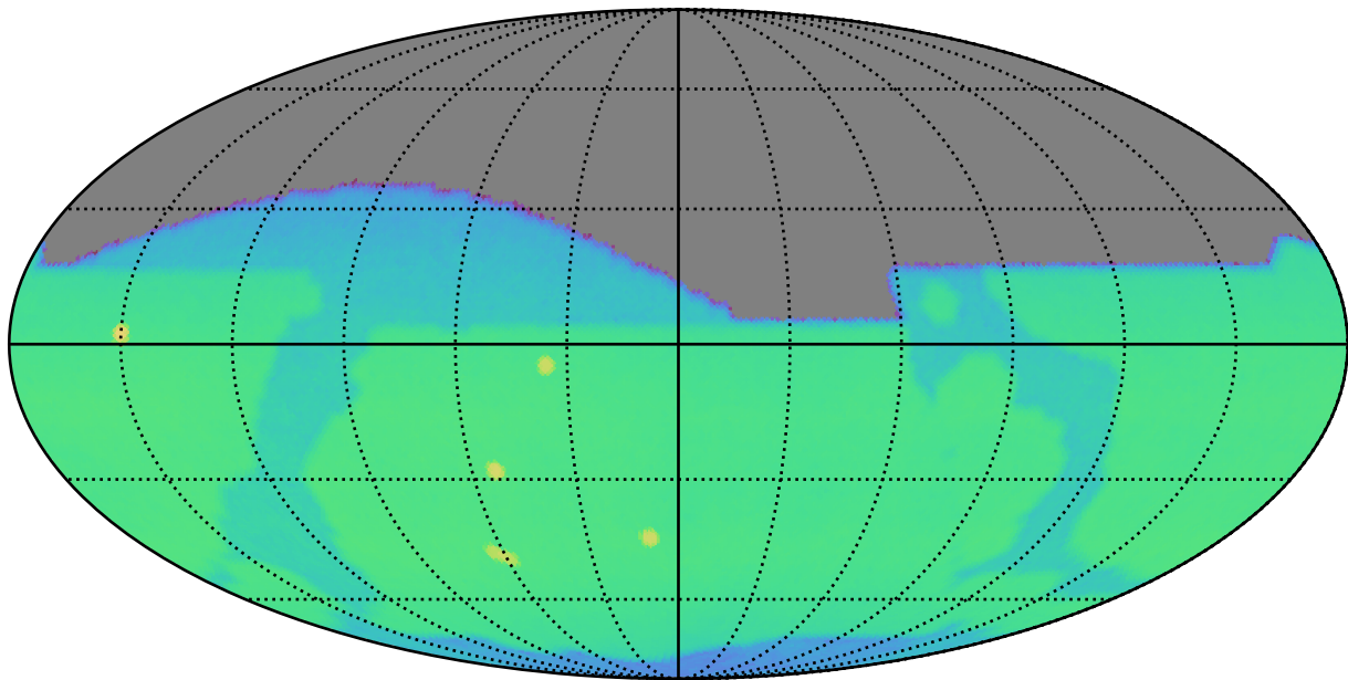
too_ignore_5_1v3.4_10yrs i: CoaddM5
