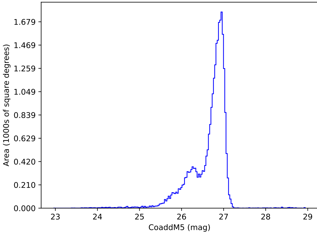
too_ignore_5_1v3.4_10yrs g: CoaddM5
