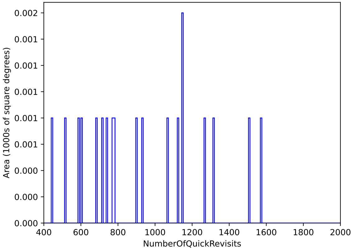
too_ignore_10_4v3.4_10yrs : NumberOfQuickRevisits
