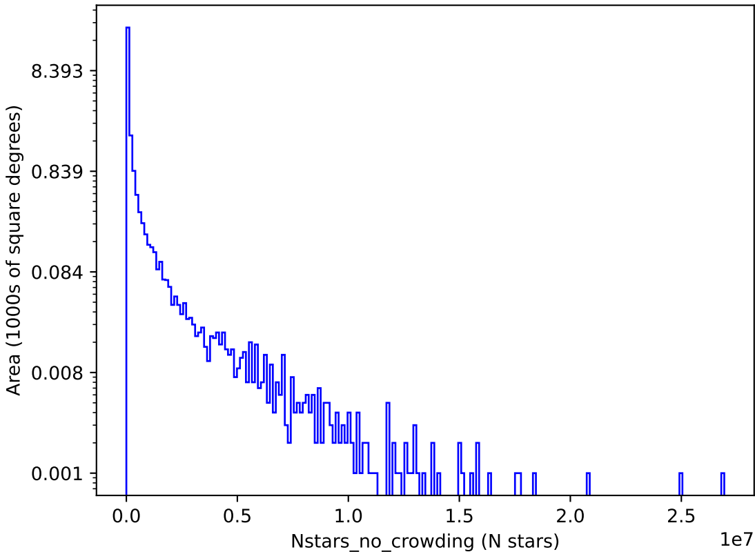
too_ignore_10_4v3.4_10yrs i: Nstars_no_crowding
