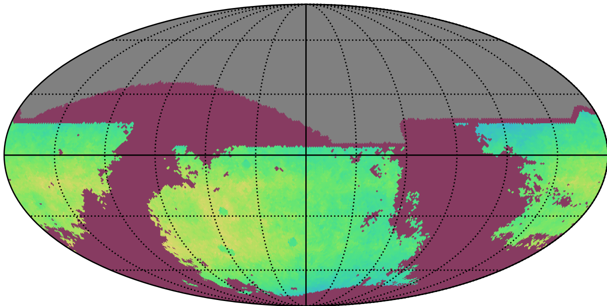
too_ignore_10_4v3.4_10yrs i: NgalScale
