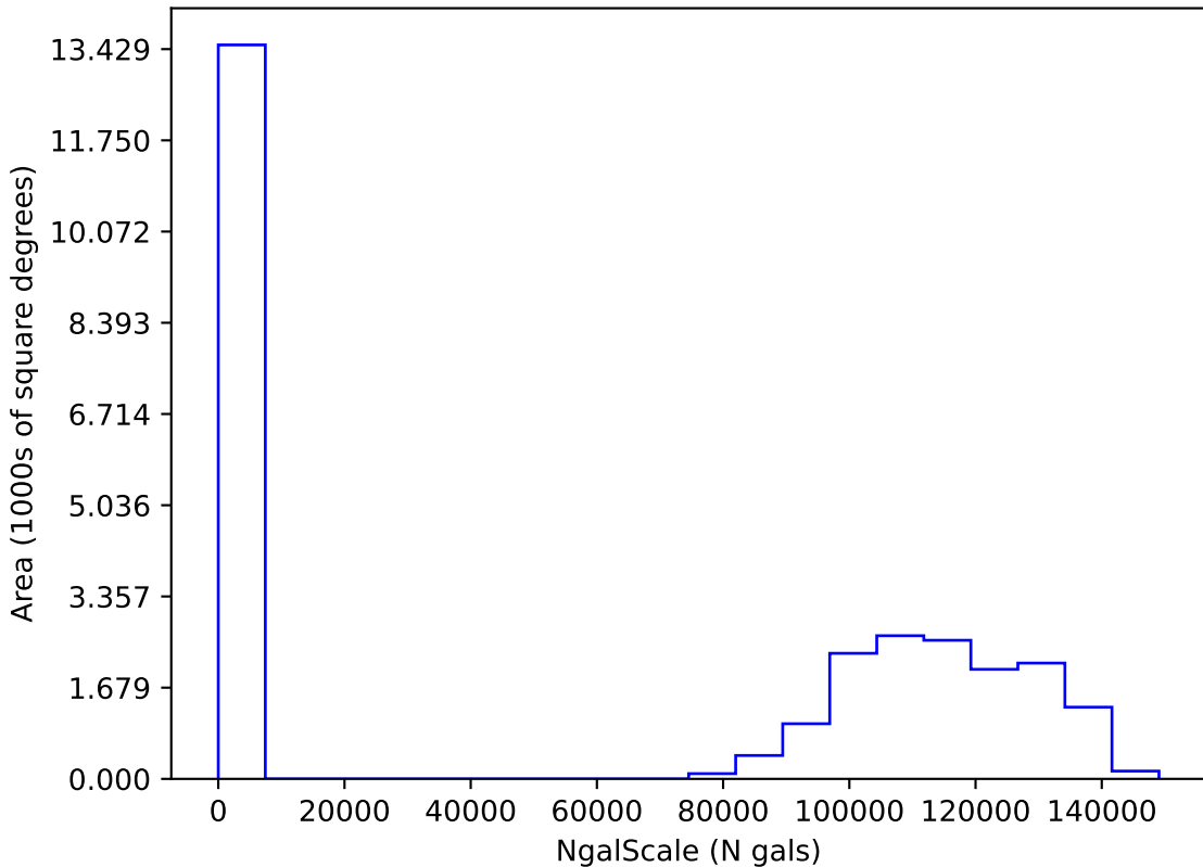
too_ignore_10_4v3.4_10yrs i: NgalScale
