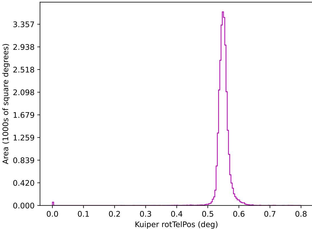
too_ignore_10_4v3.4_10yrs z: Kuiper rotTelPos
