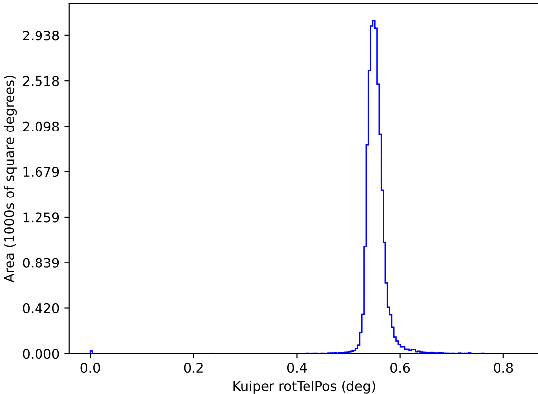
too_ignore_10_4v3.4_10yrs y: Kuiper rotTelPos
