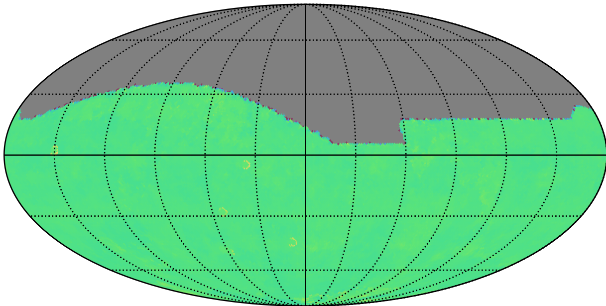
too_ignore_10_4v3.4_10yrs r: Kuiper rotTelPos
