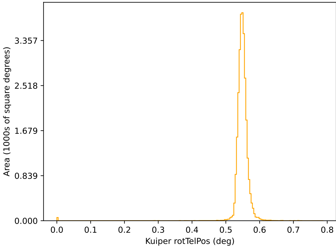
too_ignore_10_4v3.4_10yrs r: Kuiper rotTelPos
