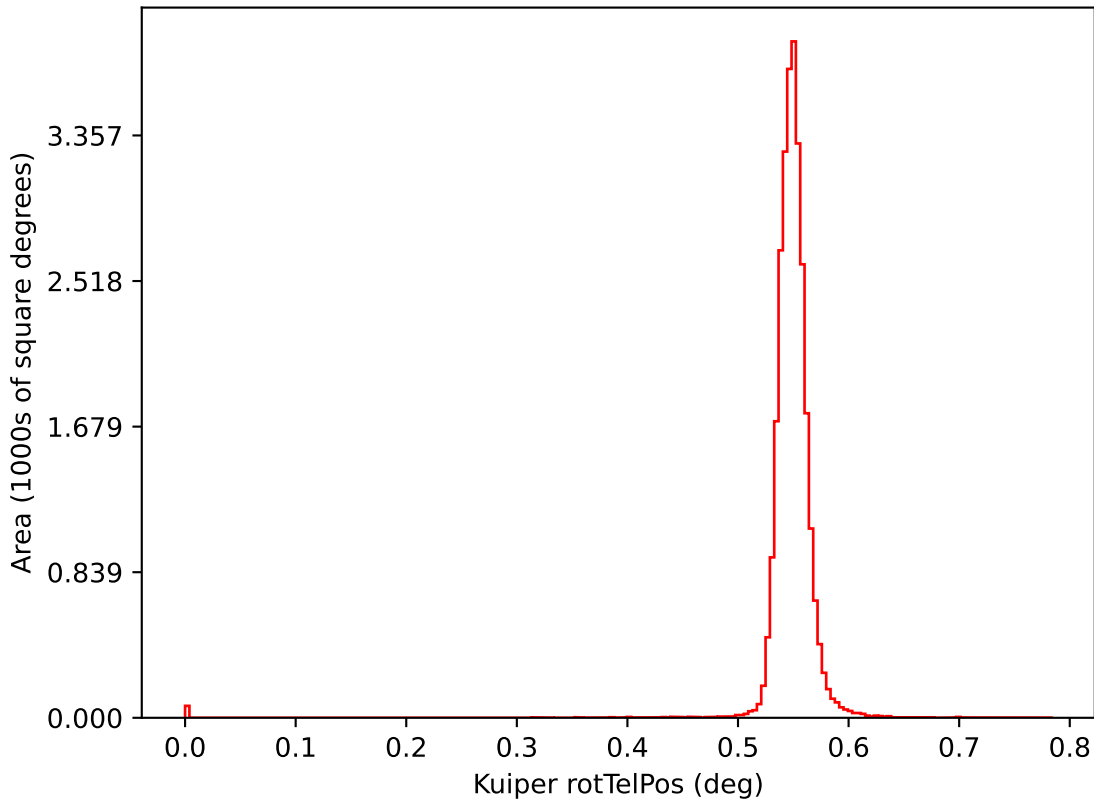
too_ignore_10_4v3.4_10yrs i: Kuiper rotTelPos
