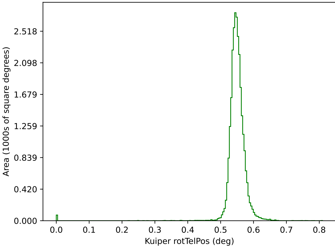
too_ignore_10_4v3.4_10yrs g: Kuiper rotTelPos
