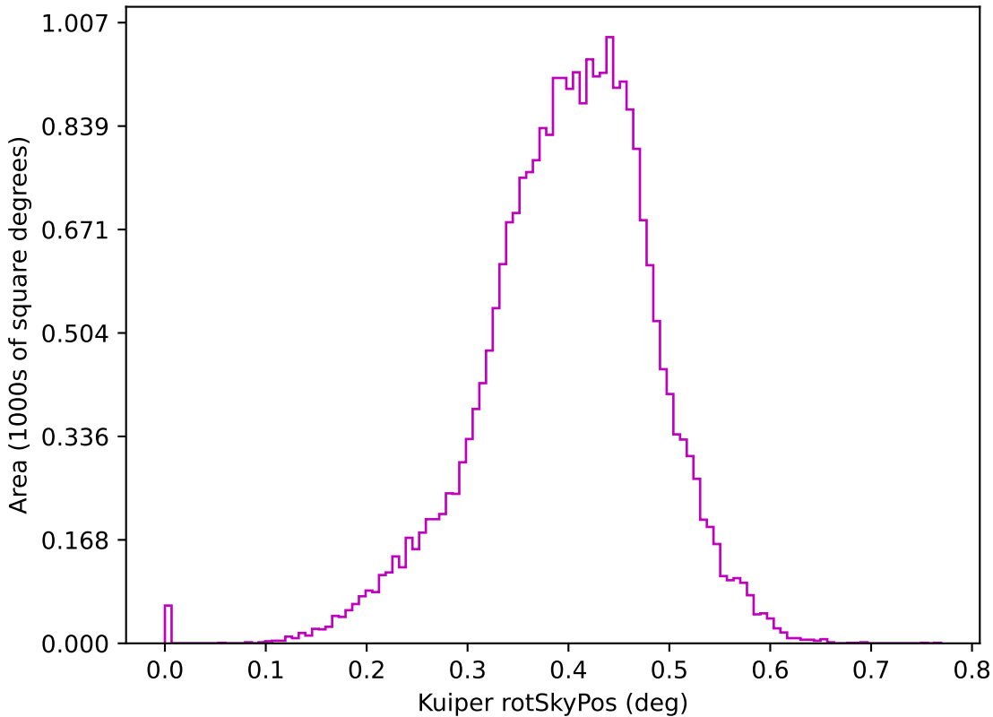
too_ignore_10_4v3.4_10yrs z: Kuiper rotSkyPos
