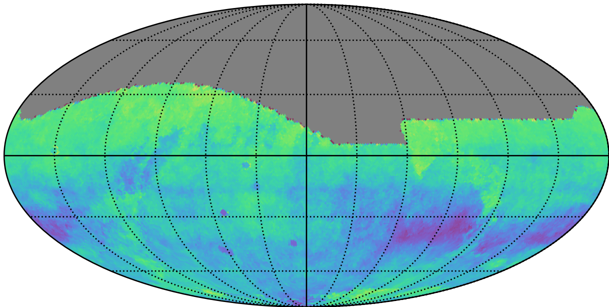
too_ignore_10_4v3.4_10yrs r: Kuiper rotSkyPos
