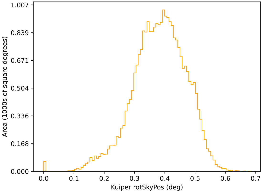
too_ignore_10_4v3.4_10yrs r: Kuiper rotSkyPos
