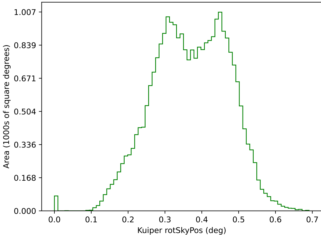
too_ignore_10_4v3.4_10yrs g: Kuiper rotSkyPos
