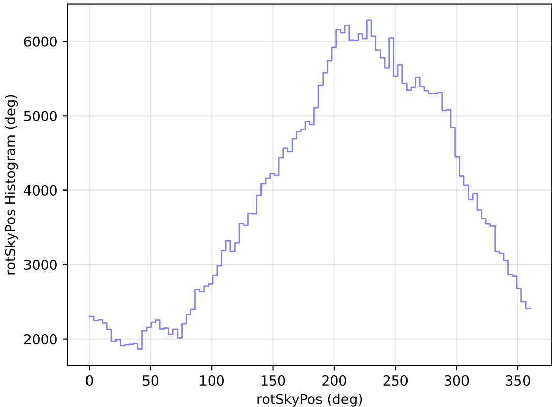
too_ignore_10_4v3.4_10yrs WFD y band: rotSkyPos Histogram
