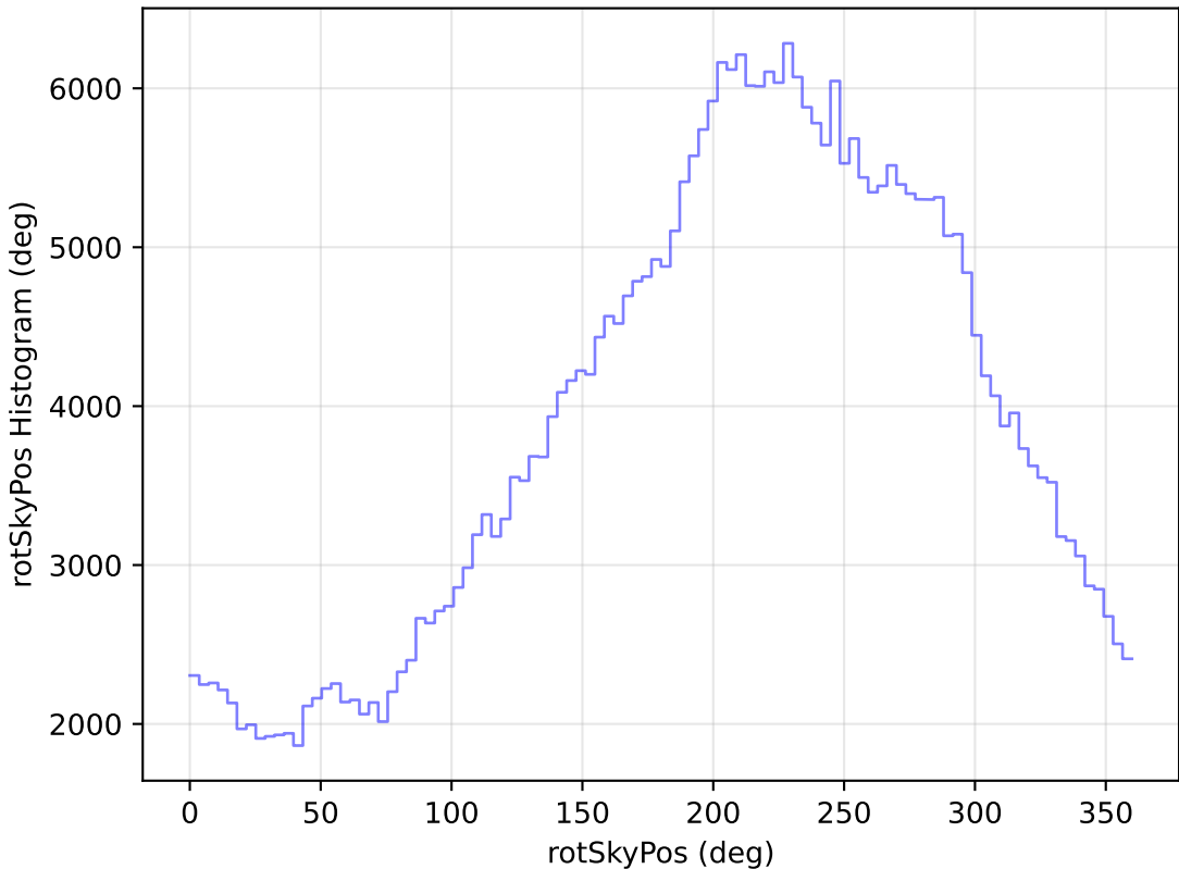
too_ignore_10_4v3.4_10yrs All sky y band: rotSkyPos Histogram
