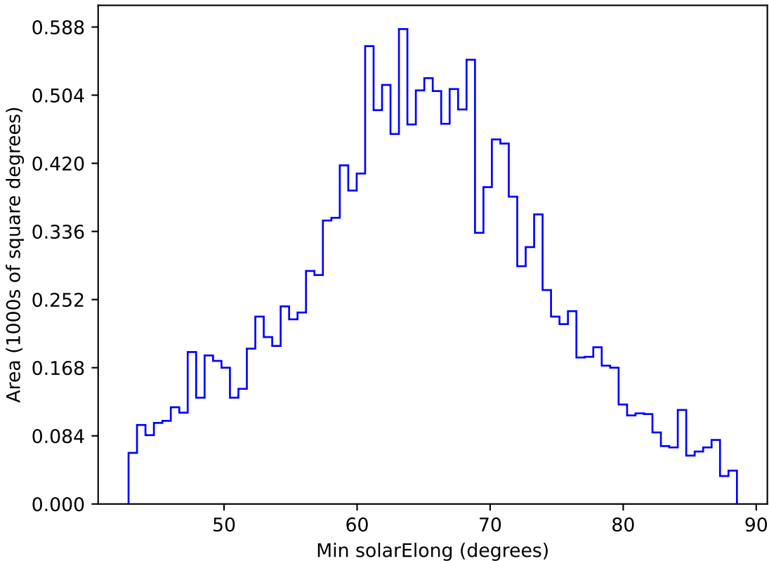
too_ignore_10_4v3.4_10yrs WFD y band: Min solarElong
