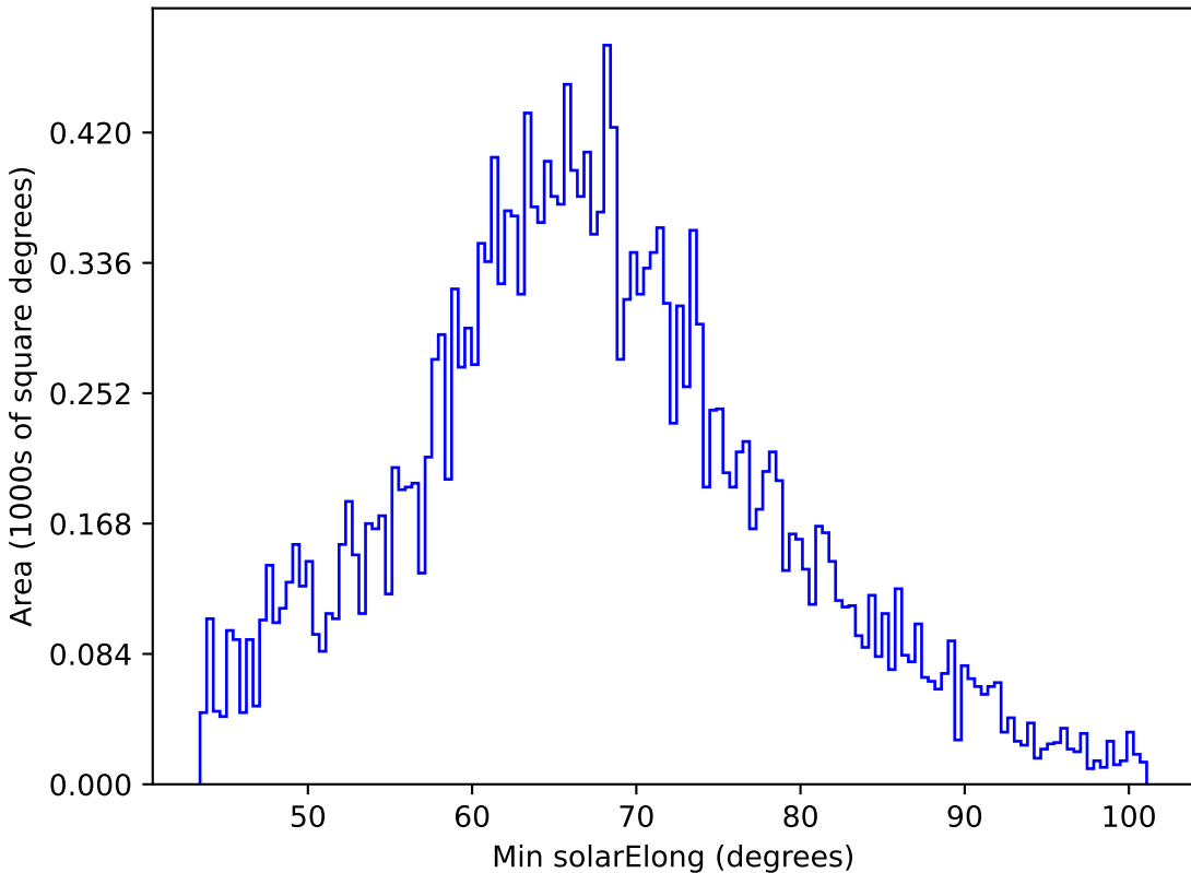
too_ignore_10_4v3.4_10yrs All sky y band: Min solarElong
