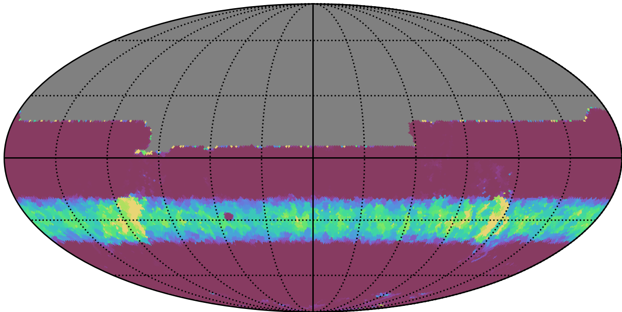
too_ignore_10_4v3.4_10yrs All sky y band: Min normairmass
