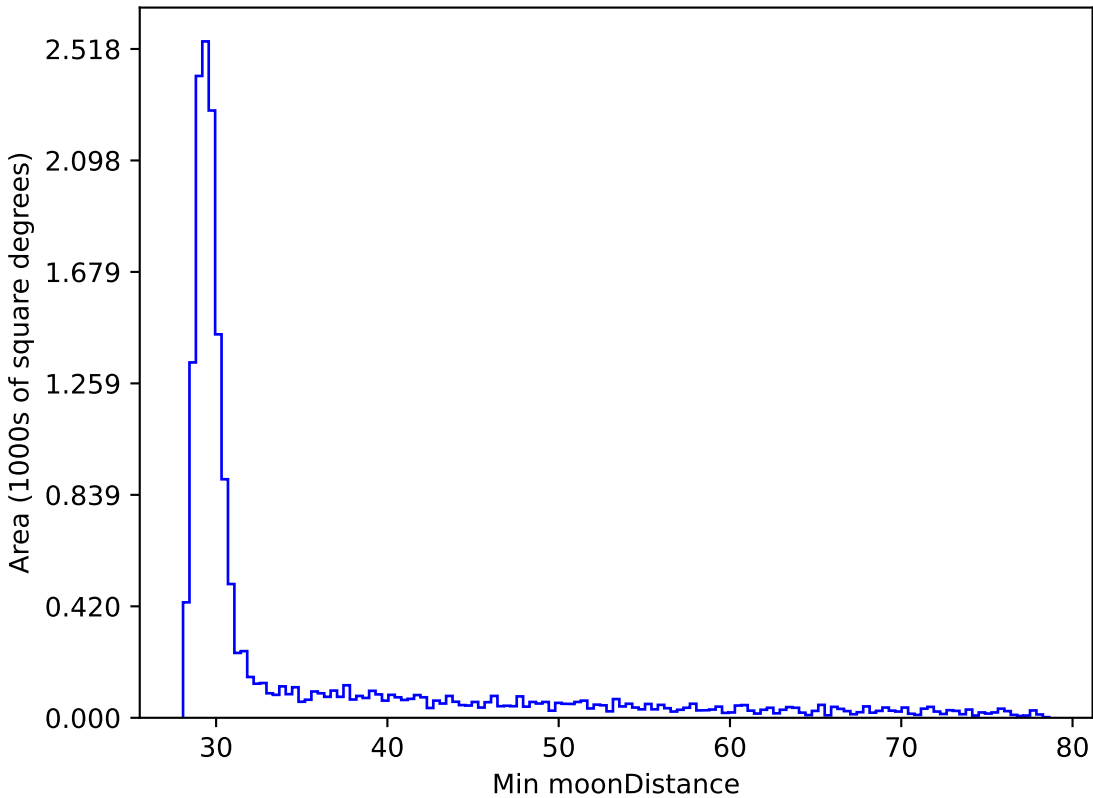
too_ignore_10_4v3.4_10yrs WFD y band: Min moonDistance
