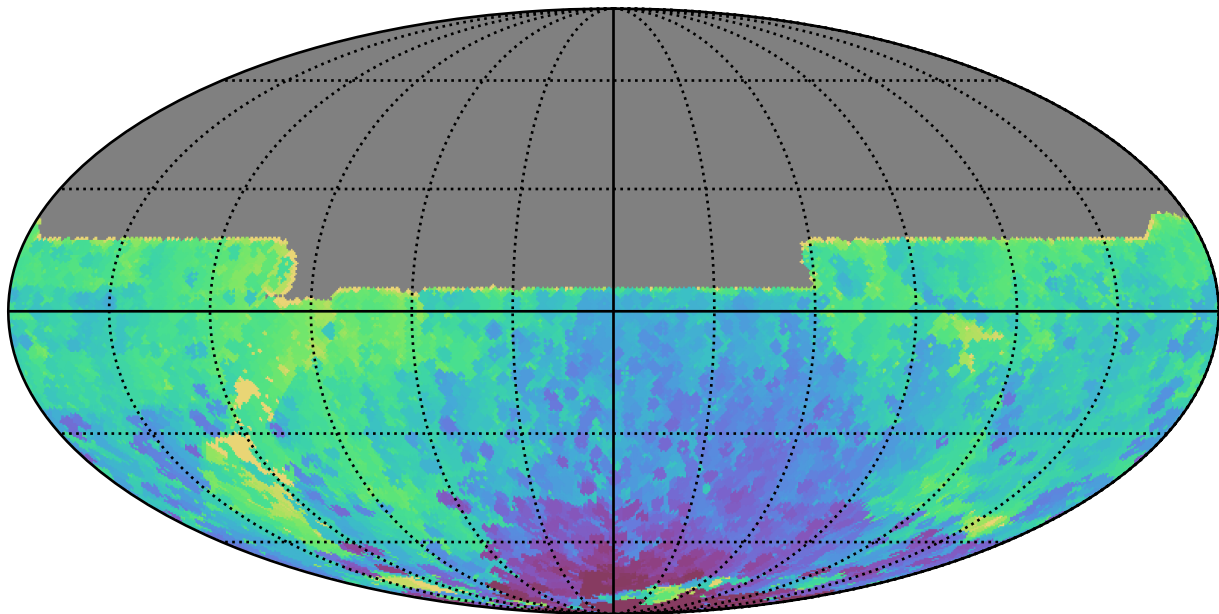
too_ignore_10_4v3.4_10yrs All sky y band: Min HA
