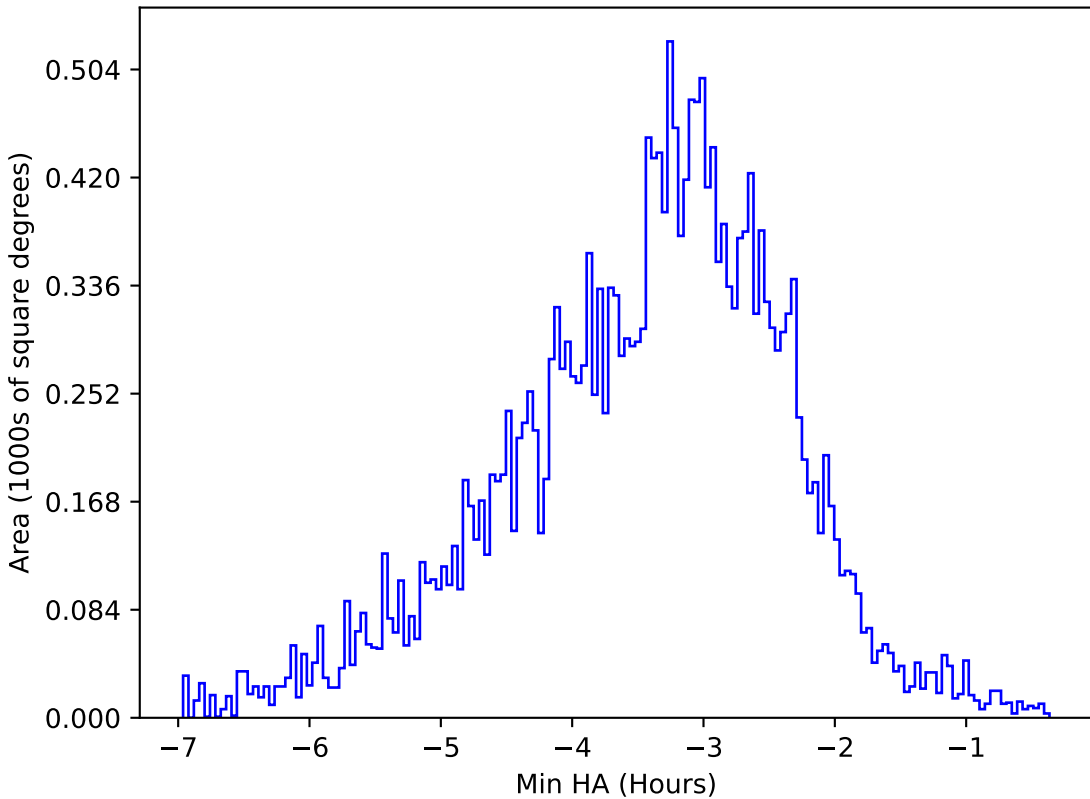
too_ignore_10_4v3.4_10yrs All sky y band: Min HA
