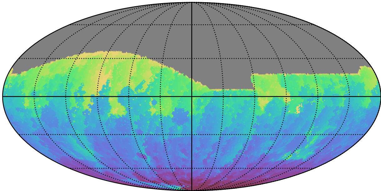
too_ignore_10_4v3.4_10yrs All sky g band: Min HA
