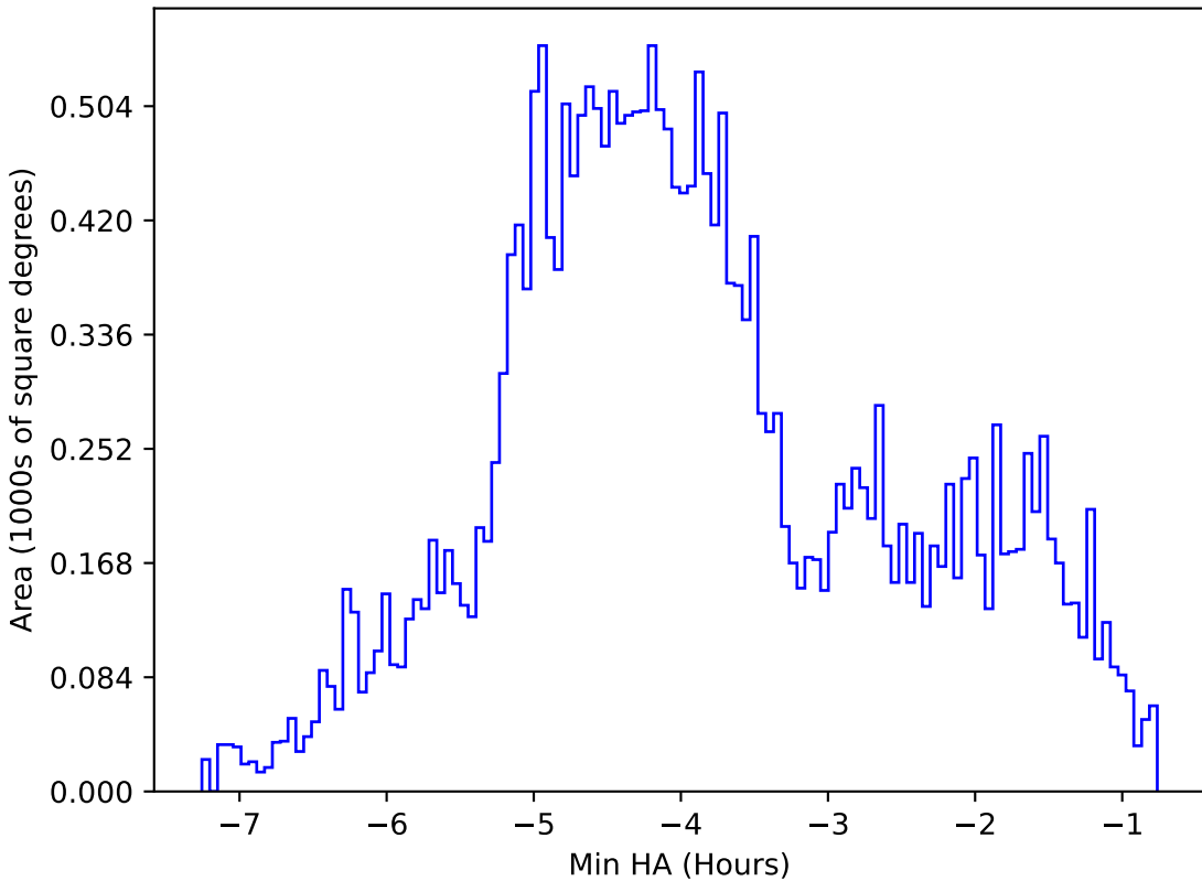
too_ignore_10_4v3.4_10yrs All sky g band: Min HA
