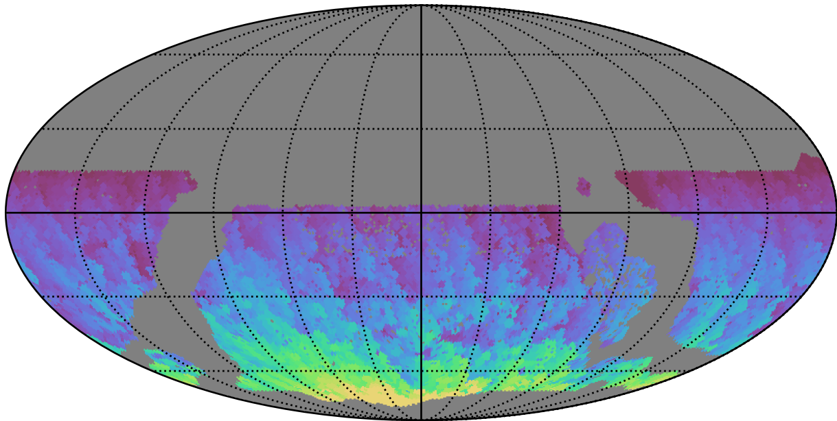
too_ignore_10_4v3.4_10yrs WFD y band: Max HA
