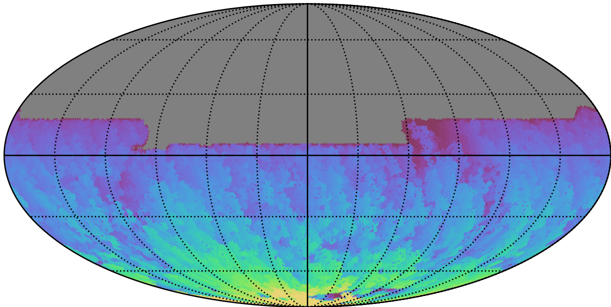
too_ignore_10_4v3.4_10yrs All sky y band: Max HA
